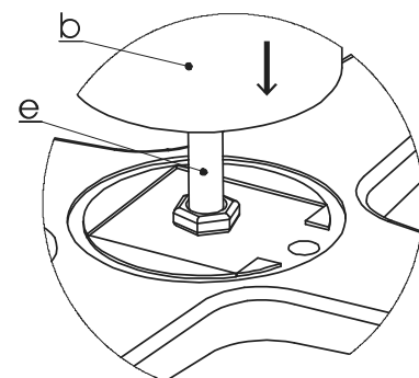
DETAIL 2.1a
